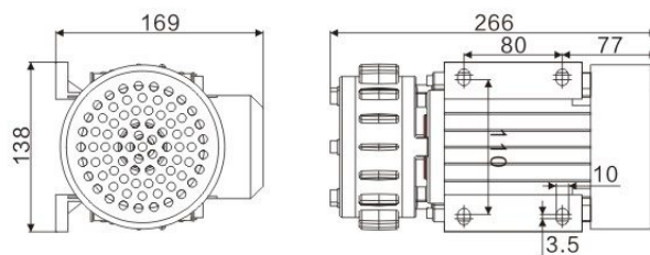
KV8尺寸图
