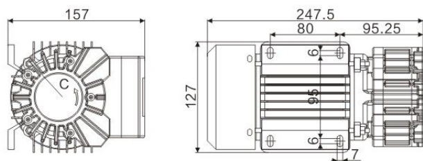
KV4尺寸图
